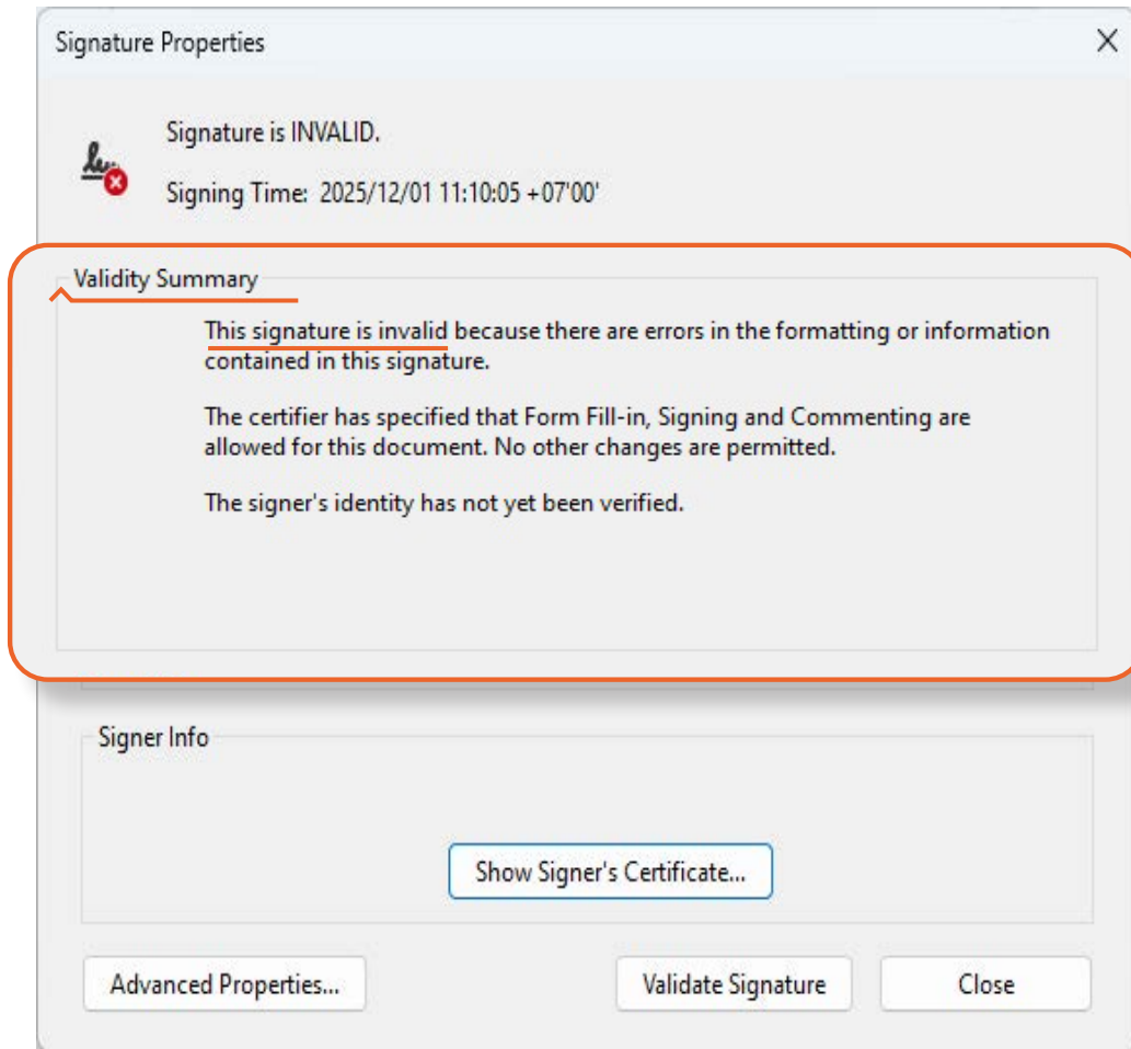
รูปที่ 13 ตัวอย่างภาพ หน้าต่าง Signature Properties แสดงผลการตรวจสอบมือชื่อดิจิทัลไม่น่าเชื่อถือ
