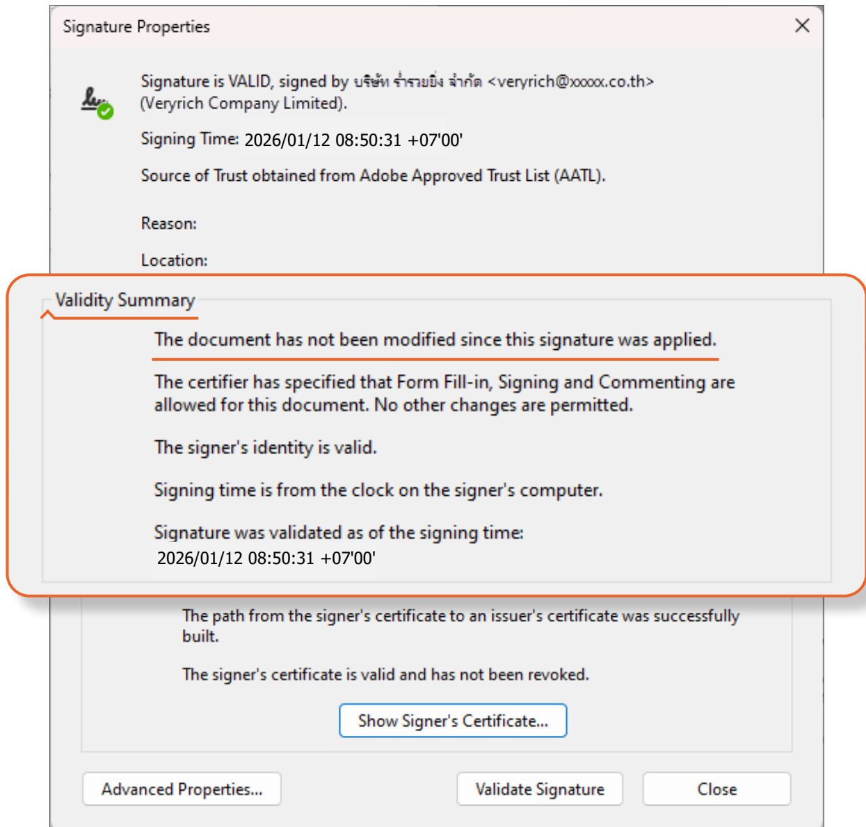
รูปที่ 9 ตัวอย่างภาพ หน้าต่าง Signature Properties แสดงผลตรวจสอบลายมือชื่อดิจิทัลไม่พบการเปลี่ยนแปลงแก้ไข
