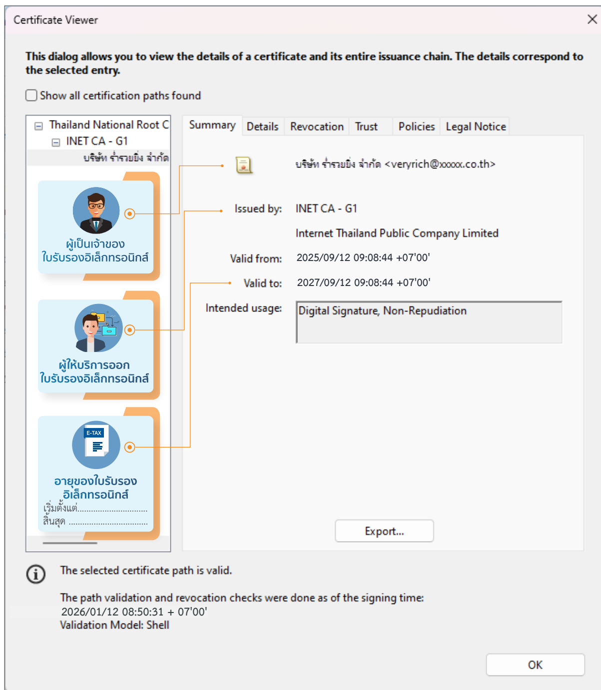
รูปที่ 11 หน้าต่าง Certificate Viewer แสดงข้อมูลใบรับรองอิเล็กทรอนิกส์ที่ใช้งาน
